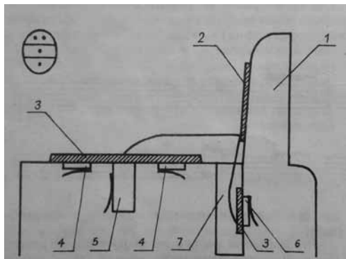
Конструкция гармони Тимофея Трофимова
